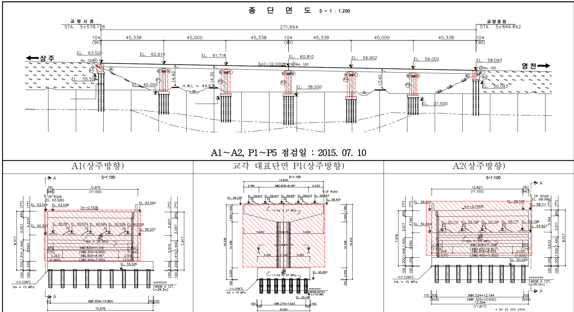
<그림 3.1> 장곡교(상주방향) 금회점검 구간 및 점검일
