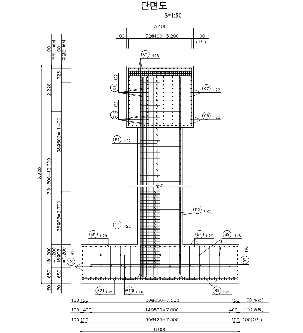
<그림 3.5> 장곡교 P3교각 배근도(영천방향)
