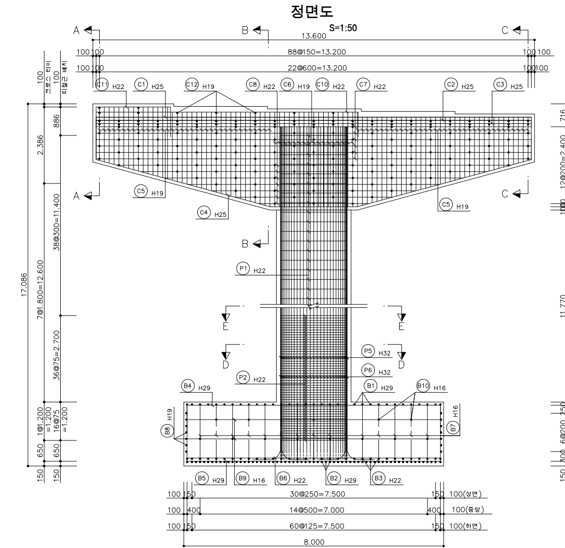
<그림 3.5> 장곡교 P3교각 배근도(영천방향)
